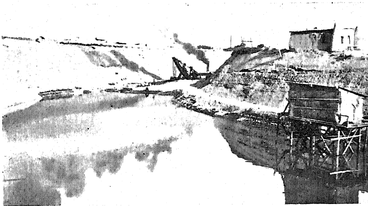
Постройка новаго канала. Вдали—экскаваторъ.
