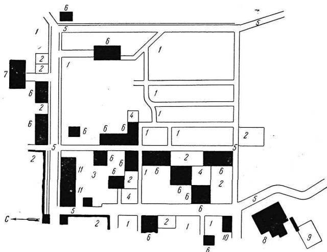
Рис. 28. Глазомерная съемка социалистического поселка колхоза им. Сталина (Кош-Куырский р-н)
