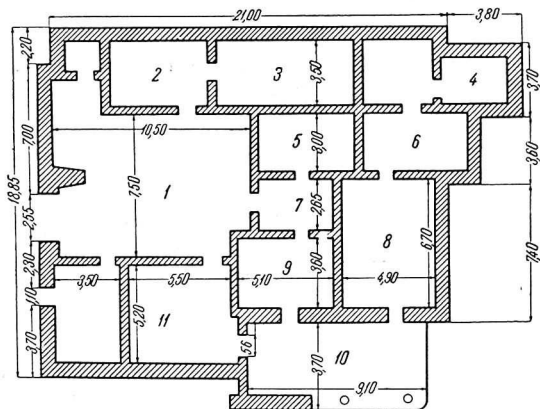
Рис. 31. План дома в колхозе им. Ахунбаева (Шабазский р-н К.-К. АССР)
