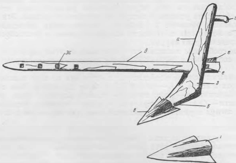
Рис. 2. Небольшой легкий омач — умочи кайроқ, сипори адир ; а — ручка омача ( даста ); б — рабочая часть омача ( нуги умоч ); в — лемех ( оҳани чурфт ); з — колышек ( дасткапак, муштак ); д — дышло ( тири умоч ); е — клинья ( фона, чи ); ж — отверстие ( тешики тири умоч ); з — комель ( кундаи умоч )
