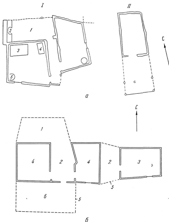
Рис. 2, а и б. Планы «там-кепбе» — построек старого типа из камыша и глины (Дарган-атинский район, аул Джигир-бент) а: I — план жилого дома; II — малятак (помещение для скота); 1 — чертен (навес из камыша); 2 — очаг; 3 — кят (деревянная кровать); 4 — стол; 5 — железная печь;
