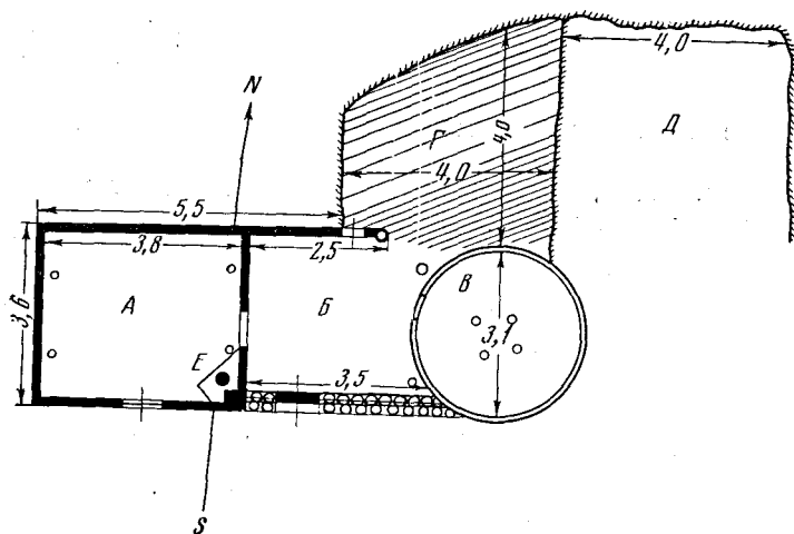
Рис. 5. Зимовка из разных строительных материалов: А — терезе или тұқпир уй — жилое помещение; Б — ағыз уй — сени и кухня; В — шошала — неподвижная юрта; Г — азбар — крытое помещение для скота; Д — құр — открытый загон для скота; Е — ошақ — очаг
