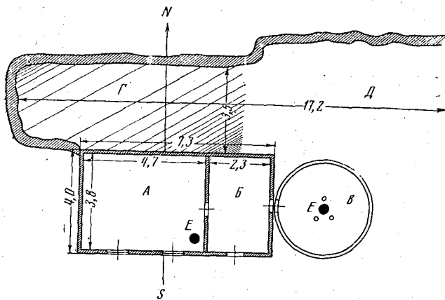
Рис. 4. Зимовка камышово-глиняная с шошала: А — терезе — жилое помещение; Б — ағыз уй — сени и кухня; В — шошала — неподвижная юрта; Г — азбар — крытое помещение для скота; Д — құр — открытый загон для скота; Е — ошақ — очаг
