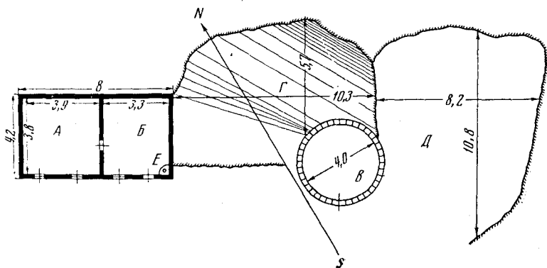
Рис. 7. Деревянная срубная зимовка с каменным фундаментом и каменная шошала: А — терезе — жилое помещение; Б — ағыз уй — сени и кухня; В — шошала — неподвижная каменная юрта; Г — азбар — крытое помещение для скота; Д — кур — открытый загон; Е — дирк — очаг
