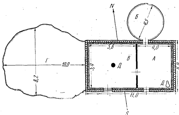
Рис. 6. Каменная зимовка: А — ағыз уй — сени, кухня; Б — шошала — неподвижная юрта; В — тұқпир уй — комната для приема гостей; Г — құр — открытый загон для скота; Д — ошақ — очаг
