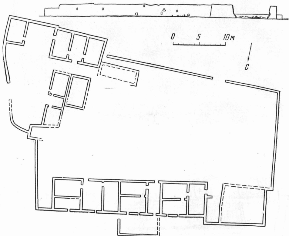
Рис. 4. План усадьбы туркмена около крепости Мангыр-Чардере (центральный район Шамурата).
