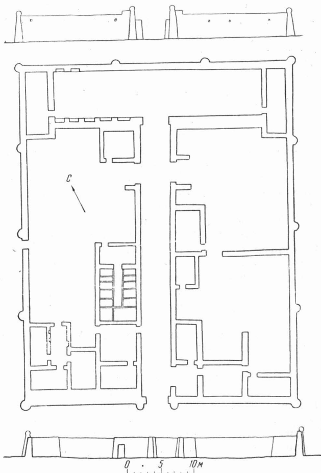
Рис. 2. Усадьба туркмена-емрели (урочище Уаз): а — главный вход; б — план усадьбы.
