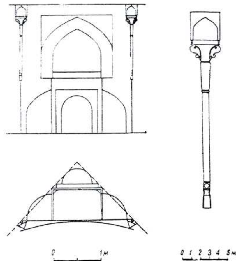
Рис. 20. Араб-ата. Паруса и колонки в интерьере.
