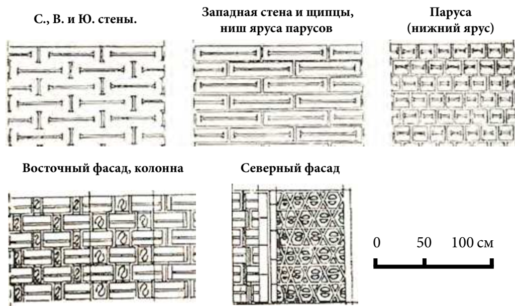
Рис. 19. Араб-ата. Кирпично-ганчевый декор мавзолея.
