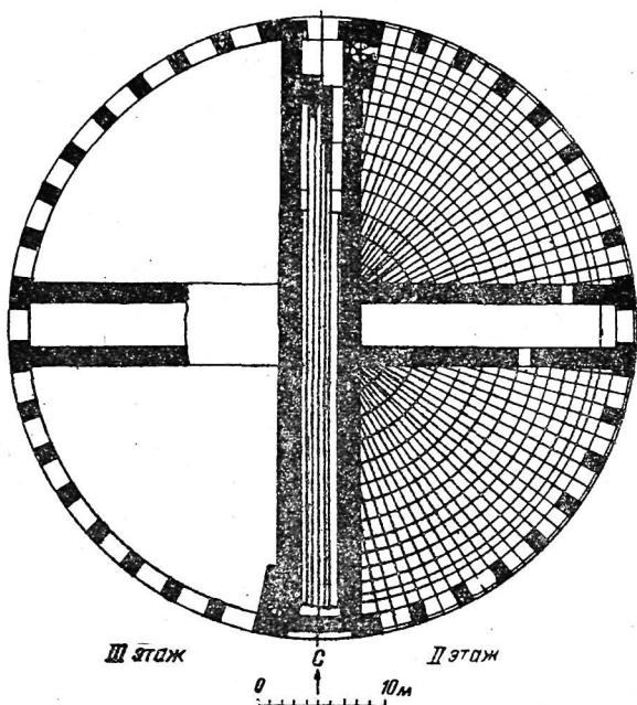
Рис. 2. План по уровням II и III ярусов.
