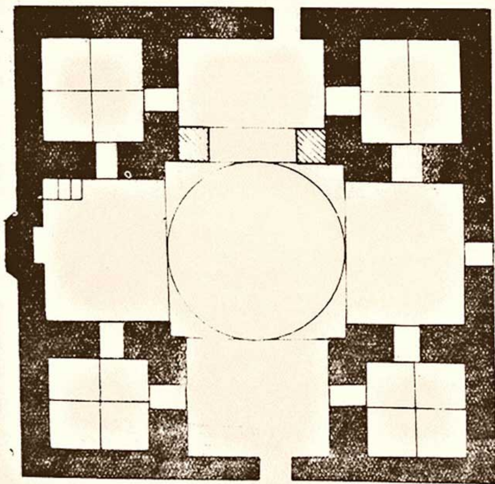
Рис. 9. Разрез и план мечети в селении Уртааул.
