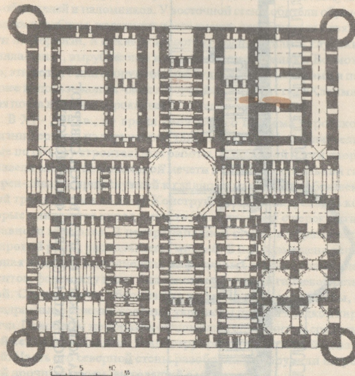
ХАНАКА КЫРК-КЫЗ. ПЛАН ПЕРЕКРЫТИЙ ПОМЕЩЕНИЙ (ПО В.М. ФИЛИМОНОВУ)
