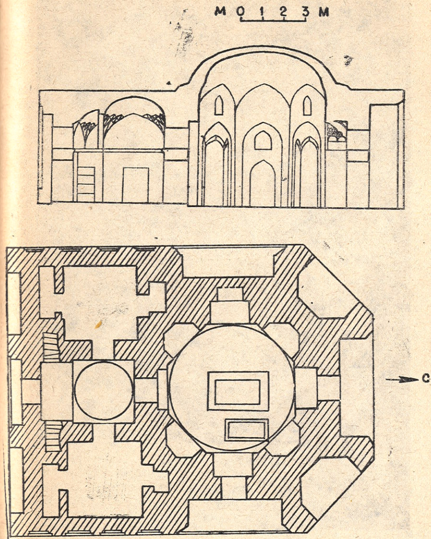
Рис. 22. План и разрез мазара Мири Рузадор (снят Г. А. Пугаченковой).
