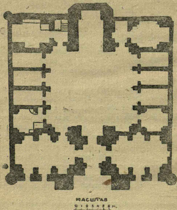
План медресе Улугбека в Гиждуване.
