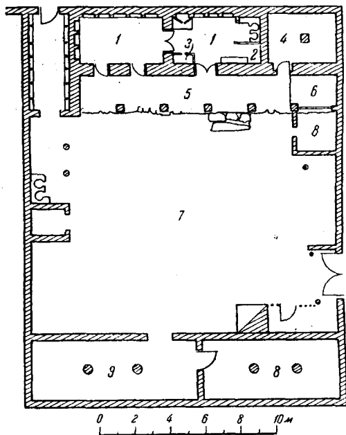
Рис. 12. Дом в Муса-базаре. План: 1 — хона; 2 — тохир хона; 3 — бугдай (амбар); 4 — угун-хона (место хранения дров); 5 — айван; 6 — тахона; 7 — ашхона; 8 — молхона (хлев); 9 — атхона (конюшня)
