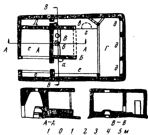
Рис. 4. План и разрезы восточного варианта позднего традиционного жилища. Дом Рахматулаева Х., к. Маргиб (Фан); А — веранда — айвон, Б — прихожая — кучаги; В — очажное отделение — мури; Г — чистое отделение — пасти боло; Д — кладовая — казнок; а — яма-зернохранилище — чагора; б — очаг; в — возвышение для стряпни — ошхона; г — ниша для дров в толще возвышения ошхона; д — стенные ниши — ток; е — глинобитное возвышение — суфа
