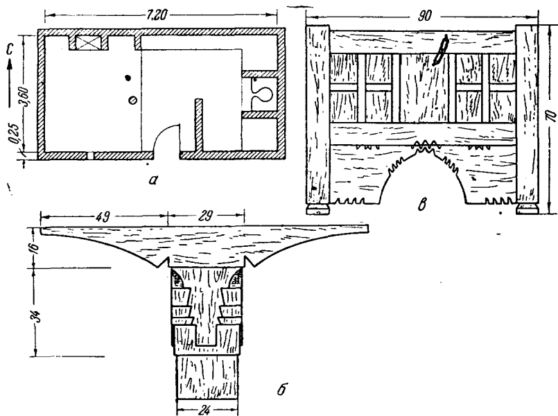
Рис. 3. Дом эмира Саида в Искондаре: а — план; б — капитель колонны; в — расписной деревянный ларь
