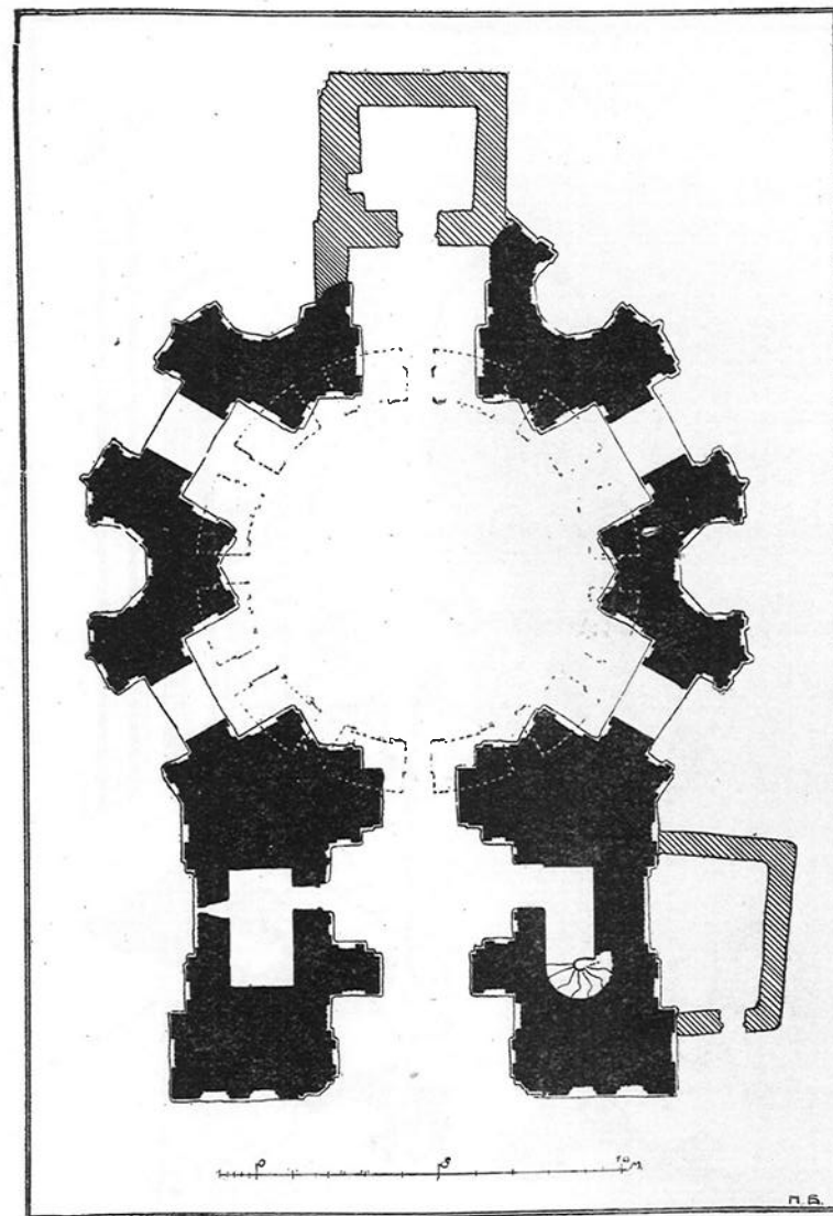
Мавзолей Тюрабек-Ханым. План.
