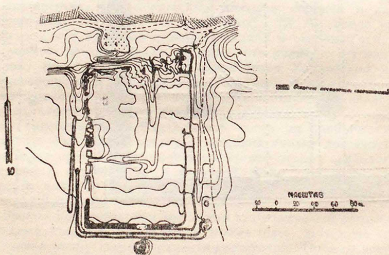
Рис. 6. План развалин крепости Хазара Составил В. А. Шишкин
