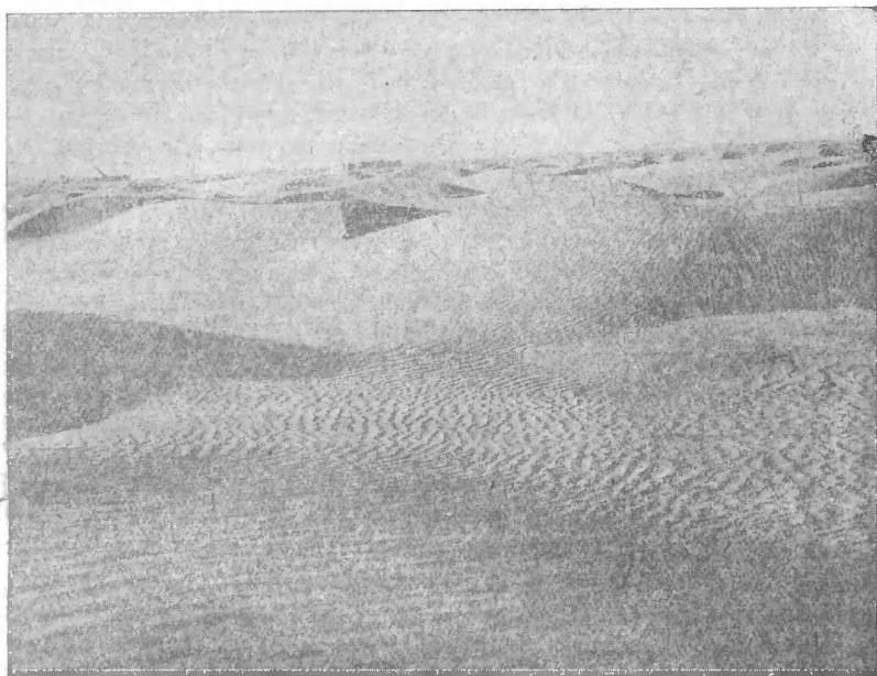
Рис. 1. Ландшафт на окраине Беркут-калинского мертвого оазиса.
