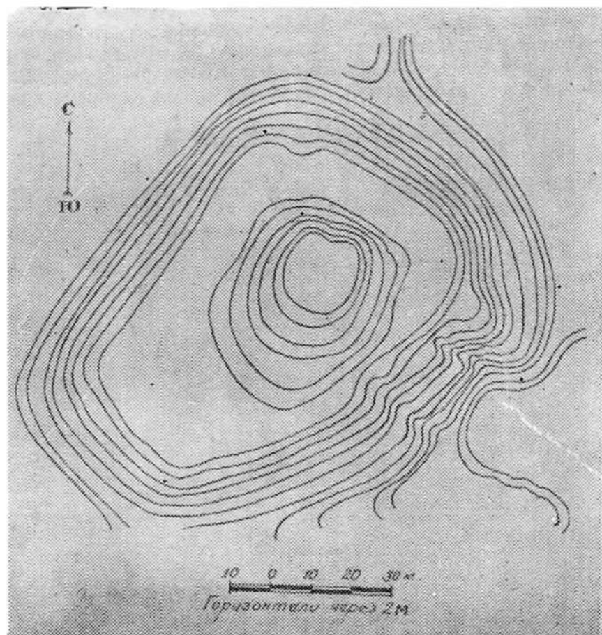
Рис. 4. Уртакурған. План холма.
