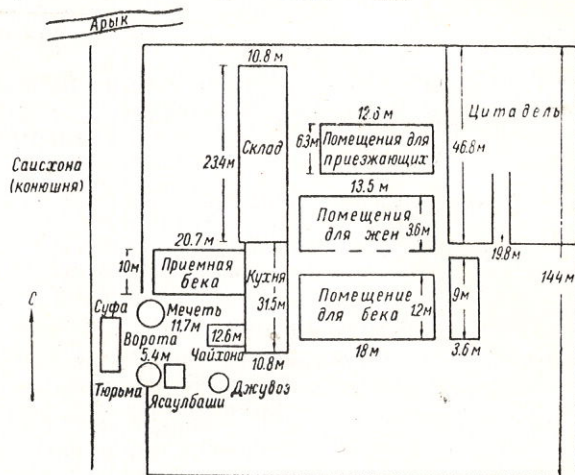
Рис. 2. Схематический план бекской крепости в Кобадияне.
