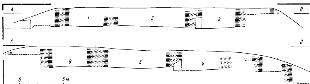
Рис. 2. Городище Билувуртепе. Разрезы через стены
