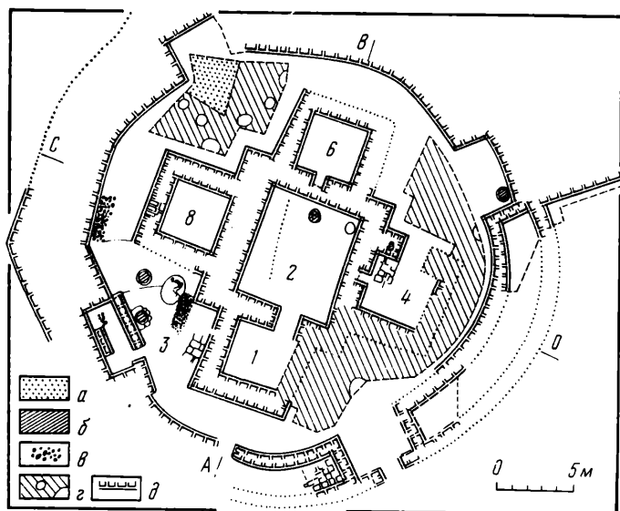
Рис. 1. Городище Билувуртепе. План цитадели
