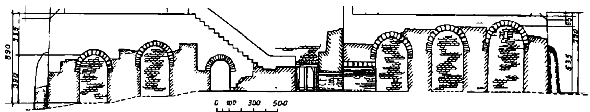
Рис. 5. Арк-тепе. Центральное здание. Разрез Г — Г. Реконструкция
