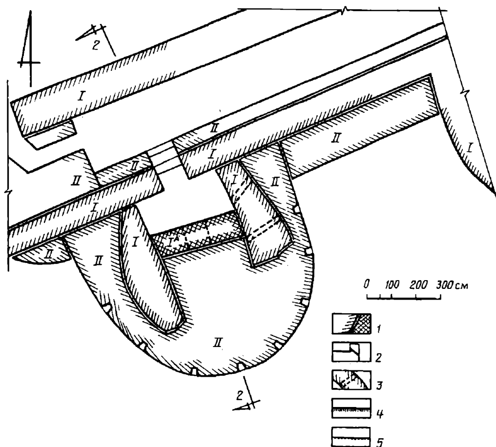
Разрез 2-2
