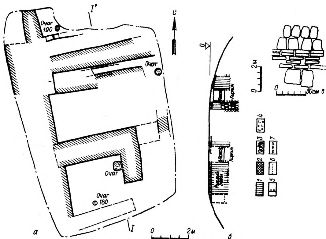
Рис. 12. Поселение 5а. План и разрез раскопа № 5. Кладка стены
