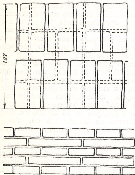
Кирпич 48-50 \times 25-27 \times 8-9
