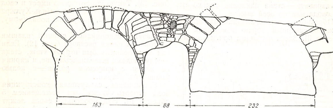
Рис. 12. Объект V. Конструкция сводов.
