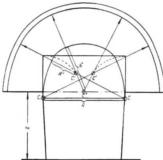
Рис. 38. Построение пятицентровой арки вала второго яруса Ак-тепе
