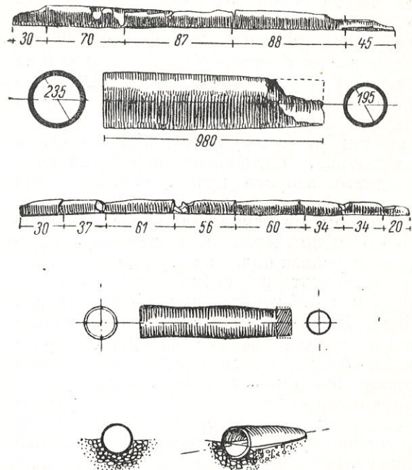
Рис. 22. Водопроводные трубы.
