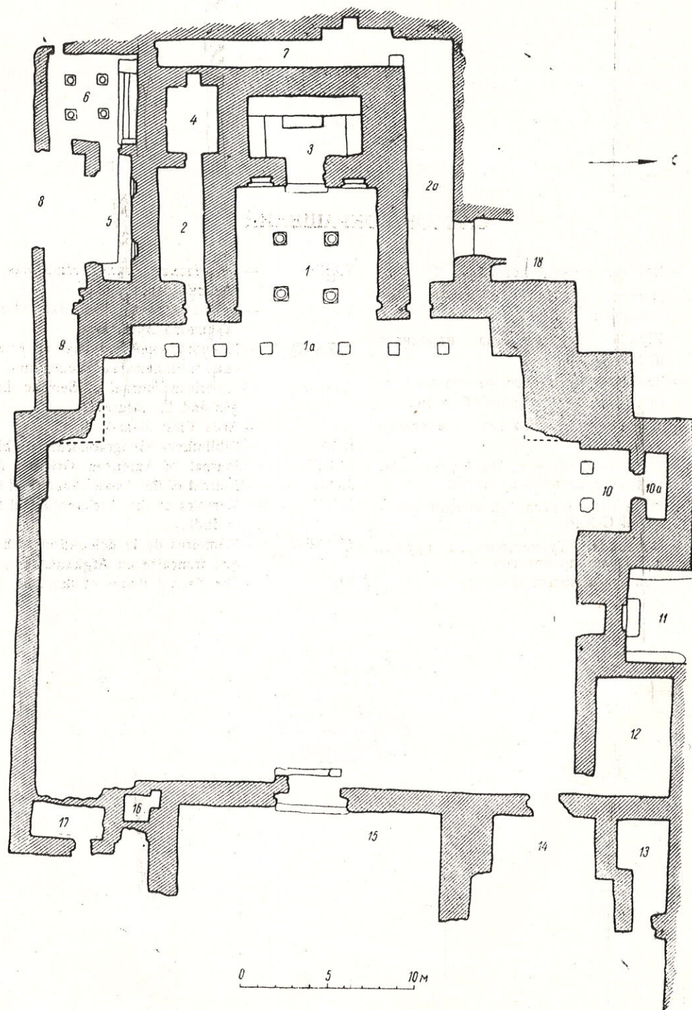
Пянджикент. План объекта I.
