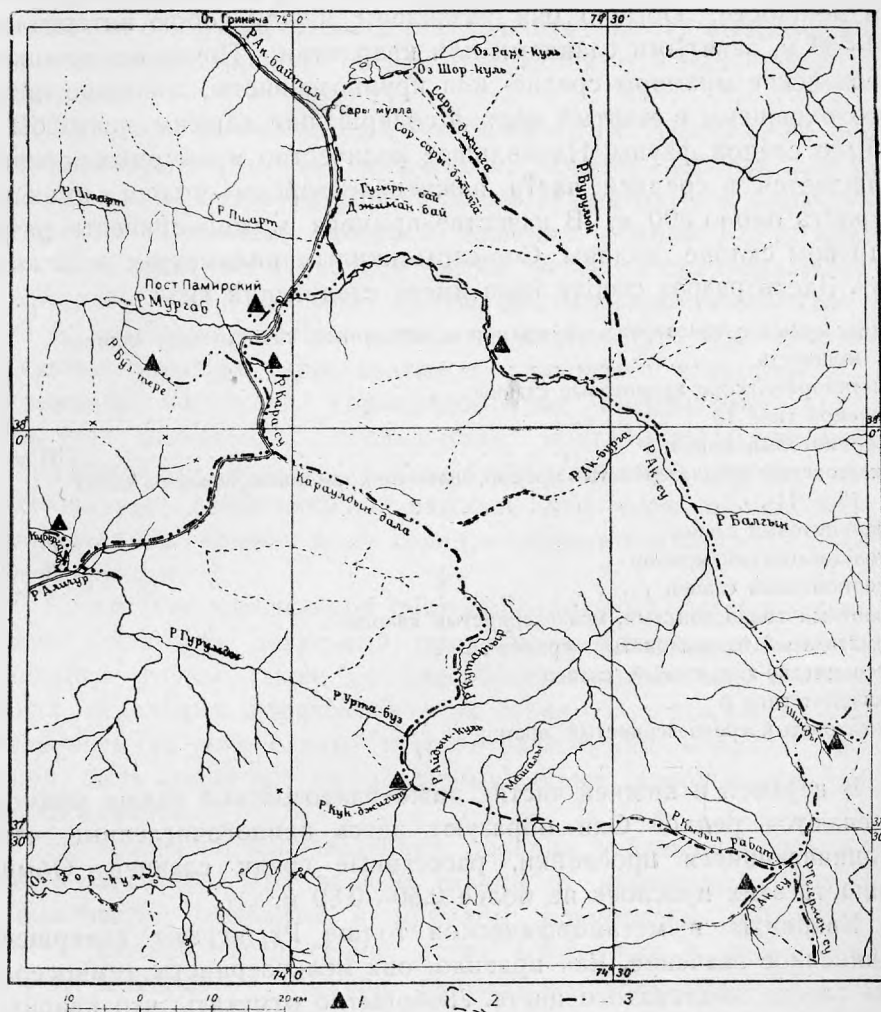
Рис. 1. Карта маршрутов и съемки Г. А. Дуткевича.
