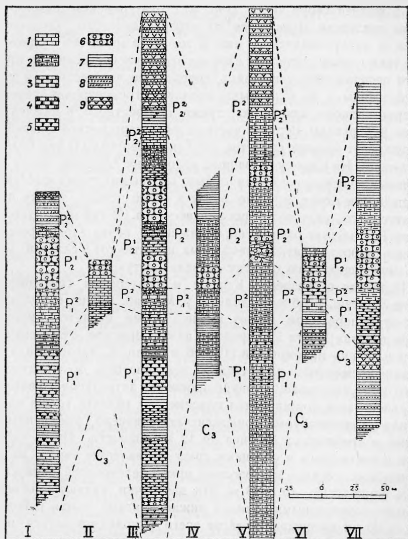
Рис. 2. Нормальные разрезы пермских отложений Восточного Памира.
