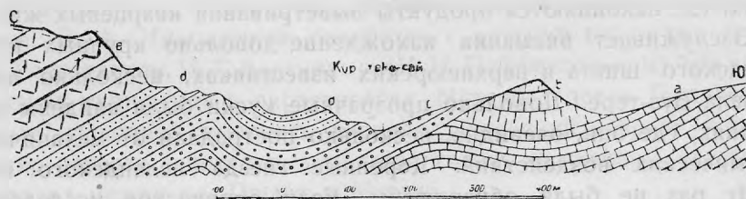
Рис. 2. Соотношение между средней и верхней юрой в верховьях Куртеке-сай.
